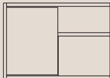
Repisa 1 W.51 H.35 D.12.4 Anclaje chazo directo
