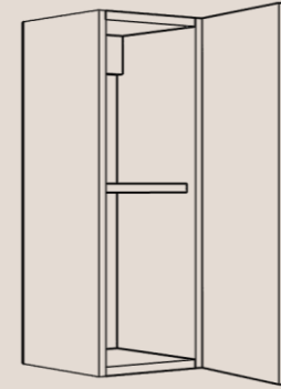
Repisa 2 W.23 H.60 D.22
